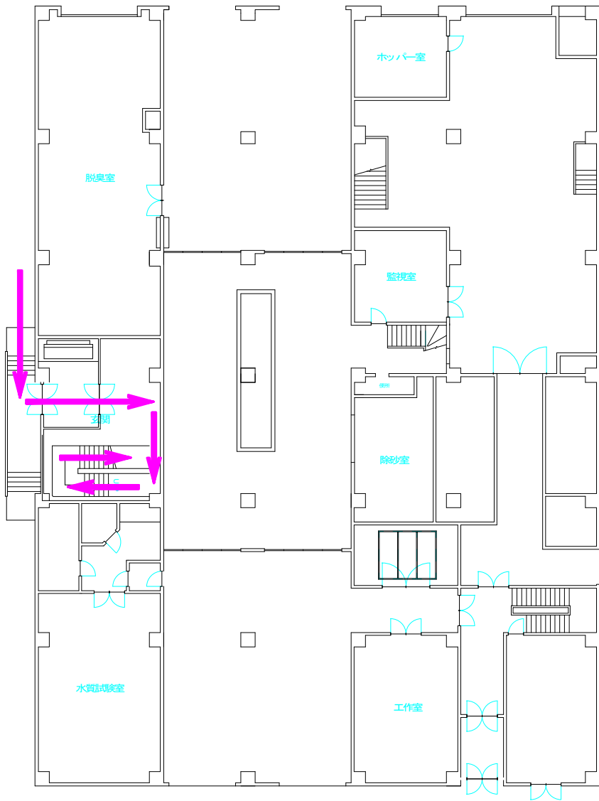
1階平面図
